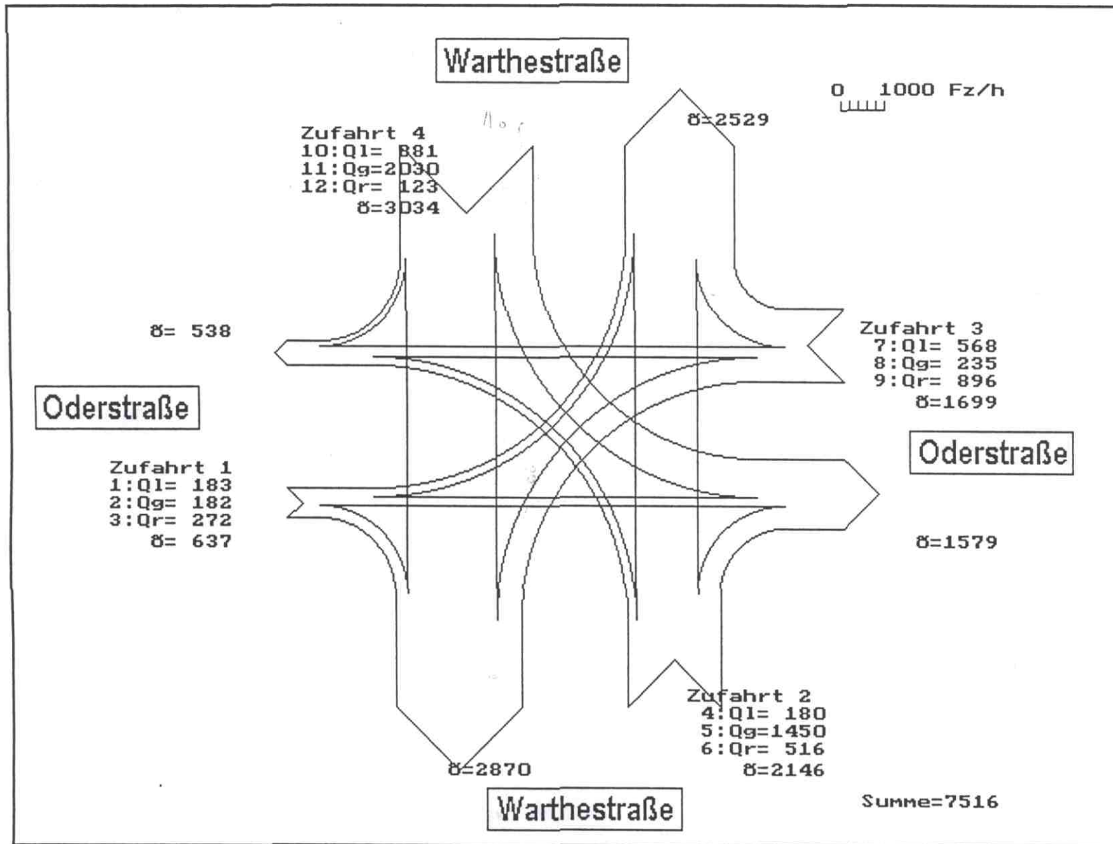
Plan 13.2: Knotenstrombelastungsplan Oderstraße/Warthestraße (Angaben in Kfz/ 4 Stunden)
